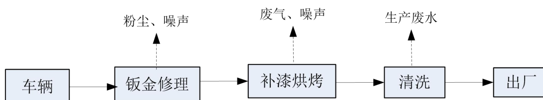
图3.5-3 项目喷漆工艺流程及其产污工艺流程图
